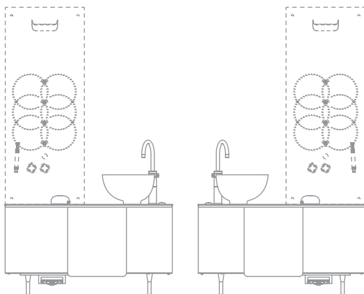
Cabinet versione sinistra Cabinet left version
